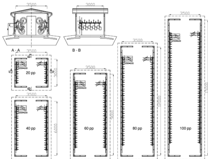
ovella® Compact PTL-2 polkupyörävarasto (tehokas pystysäilytys), leveys 3,5 metriä. Pyöräpaikat 20, 40, 60, 80 ja 100.
